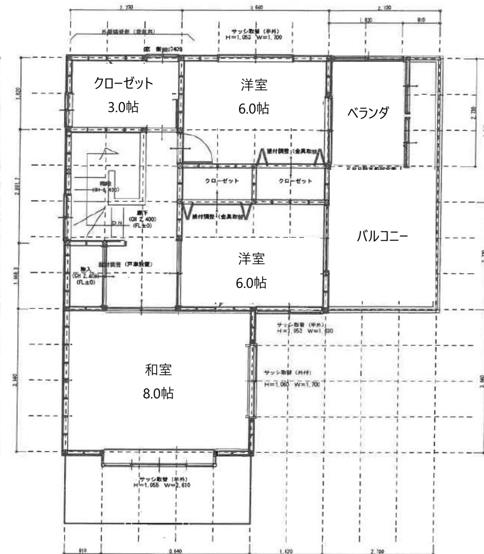
3階 平面詳細図 S:1/100
